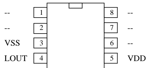
COB 管腳圖
